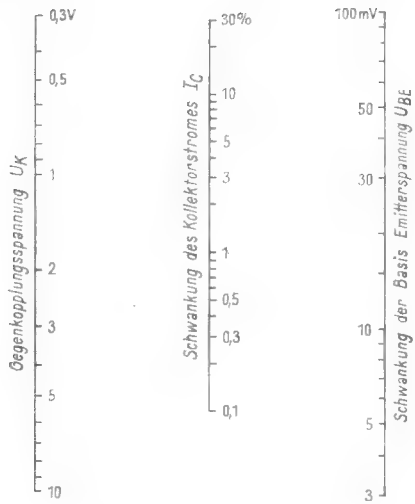
Bild 5. Die prozentualen Schwankungen des Kollektorstromes in Abhängigkeit von den Schwankungen der Basis-Emitterspannung U_{BE} und der Gegenkopplungsspannung U_K
