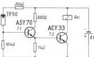
Bild 79. Lichtrelaisverstärker; das Relais zieht an, wenn die Fotodiode belichtet wird
