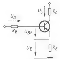
Bild 3. Die Wirkungsweise der Gegenkopplung
