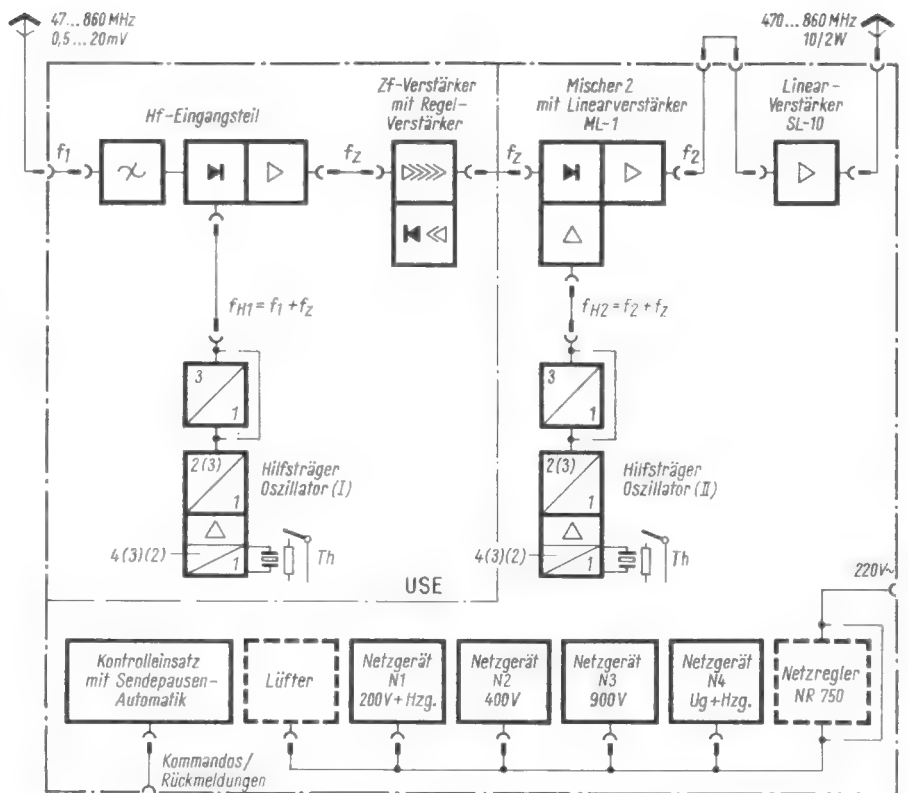
Bild 7. Blockschaltbild eines SEL-Fernseh-Frequenzumsetzers mit 10-W-Bildsender- und 2-W-Tonsender-Leistung
