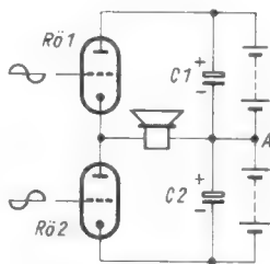
Bild 4. Die Röhre RÖ 2 und die Stromquelle sind gegenüber Bild 2 vertauscht, die Wirkungsweise ist jedoch die gleiche
