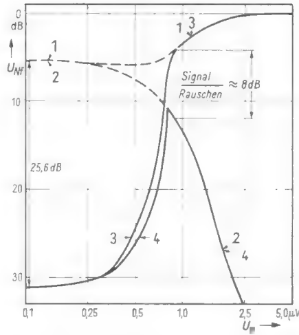
Bild 5. Dämpfungsverlauf der Rauschsperrung nach Bild 4. Bedeutung der Kurven: Nf-Ausgangsspannung ohne (1) und mit Rauschsperrung (3) bei moduliertem Signal, Rauschspannung ohne (2) und mit Rauschsperrung (4) ohne Modulation. Modulation 1 kHz, Hub \pm 15 kHz; U_B = 9 V, R_D = 8,2 k \Omega , C_{RK} = 255 pF
