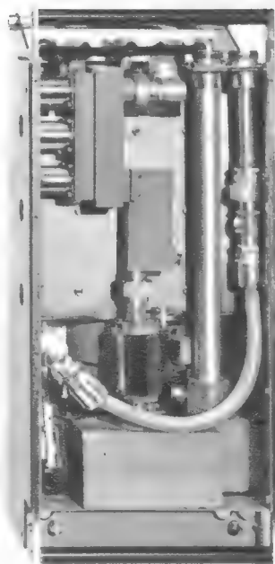
Bild 4. Parametrischer Empfangsverstärker für die Richtfunkstrecke FM 960-TV/1900 mit einer Pumpfrequenz von 6,5 GHz (Telefunken)
