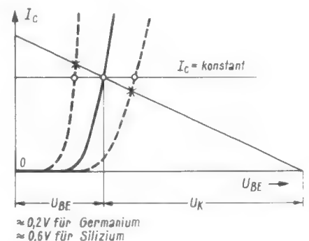
Bild 4. Einfluß der Kennlinienänderung
