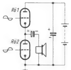
Bild 5. Aus Bild 4 entstandene Prinzipschaltung der sogenannten eisenlosen Endstufe der Philips-Geräte
