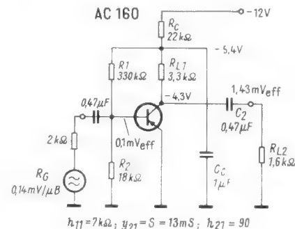
Bild 9. Mikrofonverstärker nach dem ersten Bemessungsbeispiel. Die Schaltung ist für ein magnetisches Mikrofon mit einem Innenwiderstand von 2\text{ k}\Omega ausgelegt. Zur Stabilisierung wird eine Spannungsgegenkopplung verwendet
