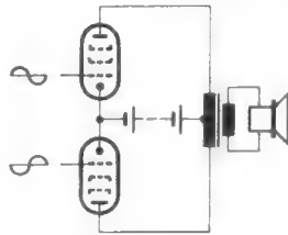
Bild 1. Herkömmliche Gegentakt-schaltung mit Ausgangsübertrager
