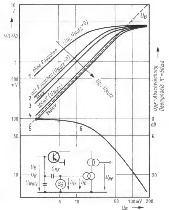
Bild 2. Dämpfungsverlauf der Rauschsperrre nach Bild 1. Die Kurven bedeuten: Nf-Ausgangsspannung ohne (1) und mit (3) Rauschsperrre bei moduliertem Signal, Rauschspannung ohne (2) und mit (4) Rauschsperrre ohne Modulation. Modulation 1 kHz, Hub \pm 15 kHz; U_B = 9 V, R_d = 8,2 k \Omega , C_{RK} = 300 pF
