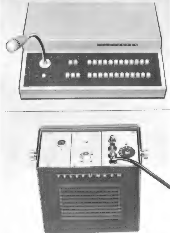
Bild 8. UKW-Personenrufanlage ELA D 600 für den Bereich 40,68 MHz. Oben: Steuergerät D 620 mit Kodiereinrichtung und Mikrofon. Unten: 5-W-Sender D 630
