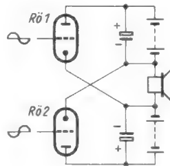
Bild 3. Durch Umzeichnen von Bild 2 entstandenes Prinzip-schaltbild des PPP-Verstärkers
