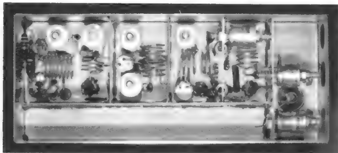
Bild 6. Aufbau des Mustergerätes
