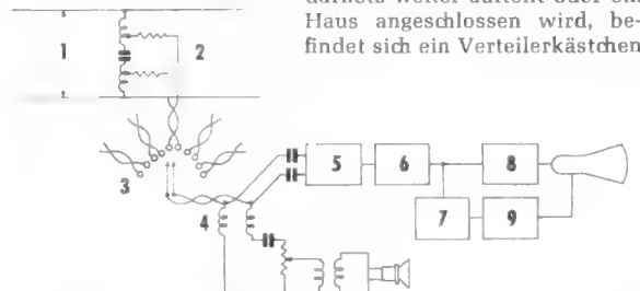
Bild 2. Teilnehmerschaltung. 1 = eine der Programmleitungen; 2 = Teilnehmer-Übertrager; 3 = Programmwähler; 4 = Hf-Drosseln; 5 = 5..11-MHz-Verstärker; 6 = Gleichrichter; 7 = Impulsabtrennung; 8 = Videoverstärker; 9 = Zeilen- und Bildablenkung mit Hochspannungserzeugung
