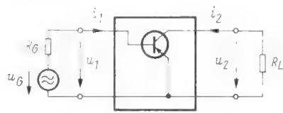
Bild 7. Wechselstromersatzschaltung einer Transistorverstärkerstufe
