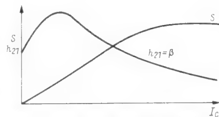
Bild 8. Verlauf von Steilheit und Stromverstärkung
