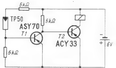
Bild 80. Das Relais fällt ab, wenn die Fotodiode belichtet wird
