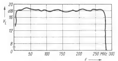
Bild 6. Frequenzverlauf im Primär-Breitband-Verteilernetz
