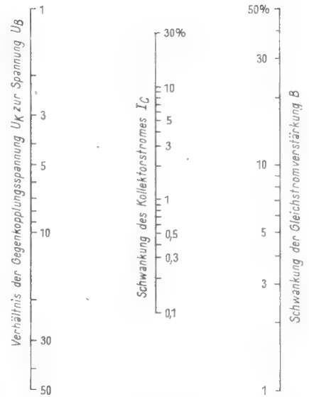
Bild 6. Die prozentualen Schwankungen des Kollektorstromes in Abhängigkeit von den prozentualen Schwankungen der Gleichstromverstärkung B und dem Verhältnis der Gegenkopplungsspannung U_K zur Spannung U_B
