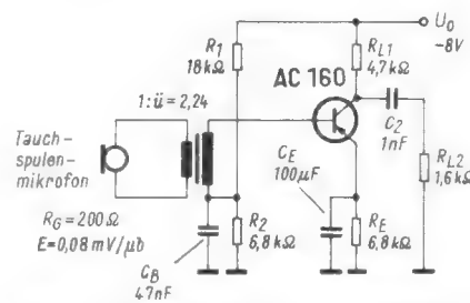
Bild 1. Schaltung eines Transistor-Mikrofonverstärkers
