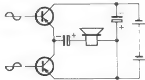
Bild 9. Transistor-Gegentaktschaltung, ähnlich der eisenlosen Endstufe nach Bild 5
