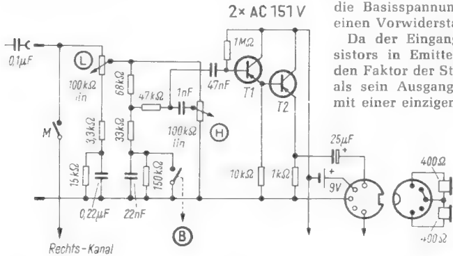
Bild 1. Schaltung des Einstell- und Anpassungsgliedes (nur für einen Kanal gezeichnet)
