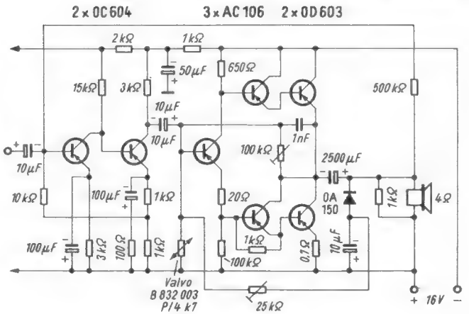
Bild 10. Schaltungsauszug eines Telefunken-Transistorverstärkers mit einer Endstufe nach Bild 9
