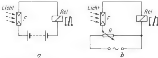
Bild 78. Einfache Lichtrelais für Batterie- und Netzbetrieb
