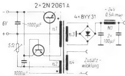
Bild 4. Schaltung des Spannungswandlers von 6 V auf 24 V. Transformator-Daten: Kern M 65/27, Dyn.-Blech IV \times 0,35 oL; n_1 = 2 \times 38 Wdg., 1,3 mm CuL; n_2 = 2 \times 42 Wdg., 0,4 mm CuL; n_3 = 200 Wdg., 0,8 mm CuL; n_4 = 8,2 Wdg./Volt
