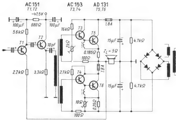
Bild 8. Schaltungsauszug einer Endstufe des Grundig-Stereoverstärkers SV 50, die nach der Grundschaltung von Bild 7 arbeitet
