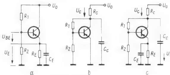
Bild 2. Stabilisierungsschaltungen; a = Stromgegenkopplung, b = Spannungsgegenkopplung, c = Strom- und Spannungsgegenkopplung
