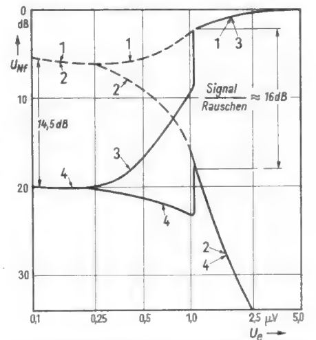
Bild 2. Dämpfungsverlauf der Rauschsperrre nach Bild 1. Die Kurven bedeuten: Nf-Ausgangsspannung ohne (1) und mit (3) Rauschsperrre bei moduliertem Signal, Rauschspannung ohne (2) und mit (4) Rauschsperrre ohne Modulation. Modulation 1 kHz, Hub \pm 15 kHz; U_B = 9 V, R_d = 8,2 k \Omega , C_{RK} = 300 pF
