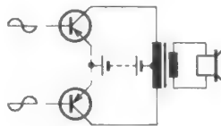
Bild 6. Transistor-Gegentakt-schaltung mit Ausgangsübertrager, die Bild 1 entspricht
