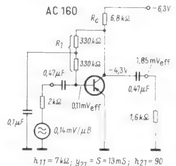
Bild 10. Abgewandelte Schaltung von Bild 9. Sie ist für kleinere Speisespannungen ausgelegt. Das Prinzip dieser Schaltung findet sich häufig in Hörgeräten
