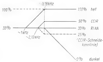
Bild 2. Stilisierte Grenzfrequenzkurven
