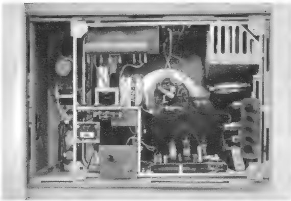
Bild 3. Rückansicht eines „Draht“-Fernsehempfängers
