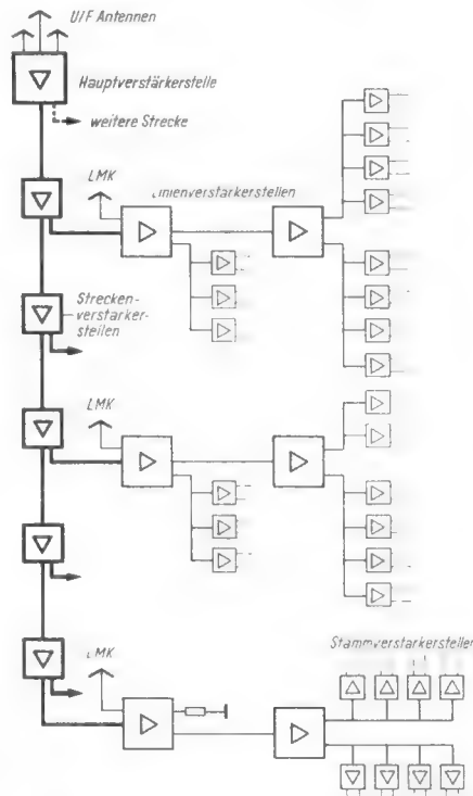
Bild 5. Prinzip einer Zentralantennen-Anlage für 1000 Teilnehmer
