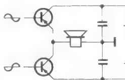
Bild 7. Transistor-Gegentakt-schaltung, die im Prinzip Bild 4 entspricht
