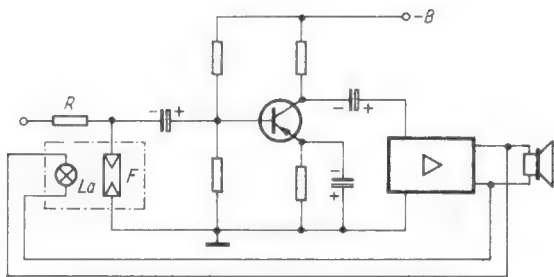
Bild 83. Fotoelektronische Dynamikregelung
